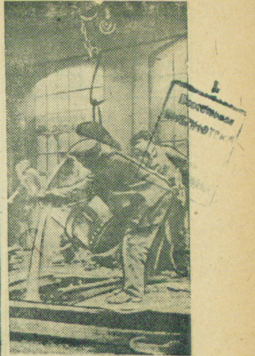
Становка покрышки для турбины в 25000 квт на зав. им. Сталина
