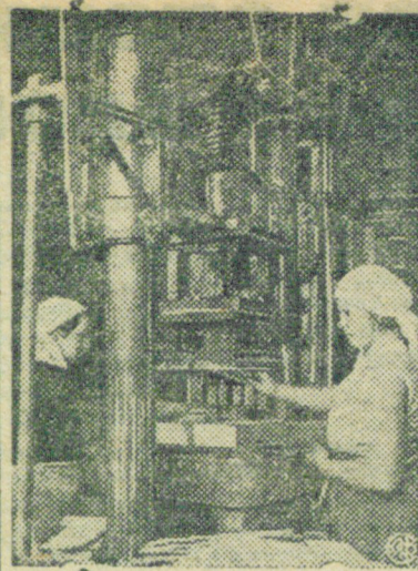
Завод „Красный Керамик“, г. Воровичи, производит огнеупорный кирпич для тяжелой промышленности. На снимке: подпрессовка огнеупорного кирпича.
