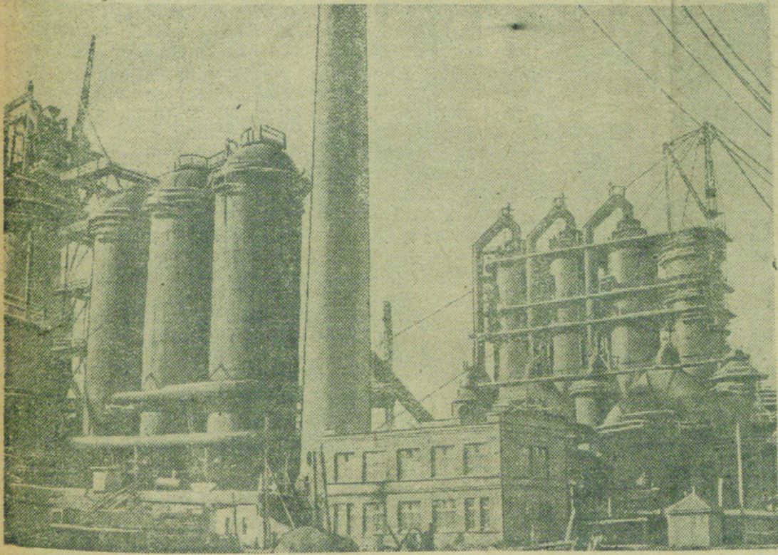
На снимке: Общий вид строительства домны № 2 (слева) и газоочистки Новотагильского металлургического завода (Свердловская область).
