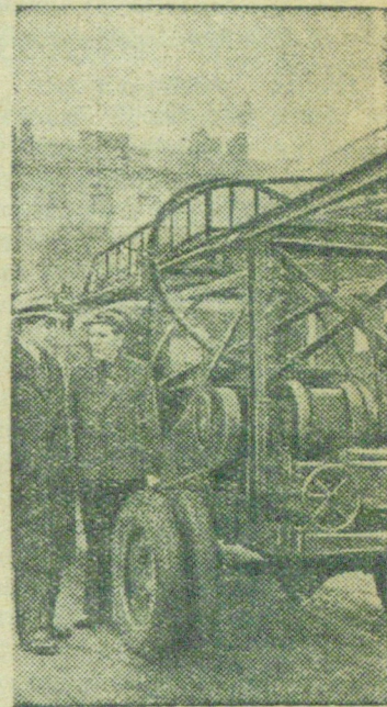
Станок „ГБГ—50“, смонтированный на грузовике. Фото В. Тарасевича. Фото ТАСС.
