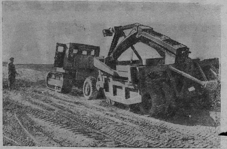
Трасса Главного Туркменского канала. От Тахиа-Таш до города Ходжейли прокладывается шоссе. На строительстве широко применяются мощные дорожные механизмы.
