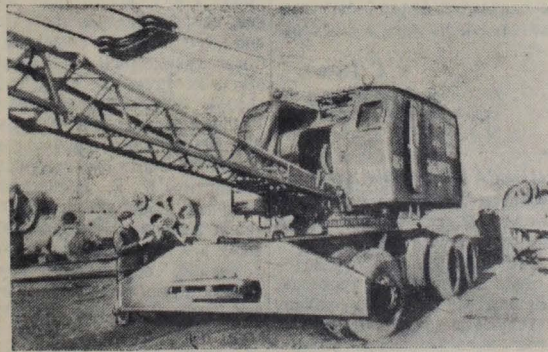
Запорожская область. В адрес «Укрводострой» прибывает мощная советская техника, которая будет использована на строительстве Южно-Украинского канала. На снимке: подъемный кран новой конструкции, прибывший с одесского завода имени Январского восстания.
