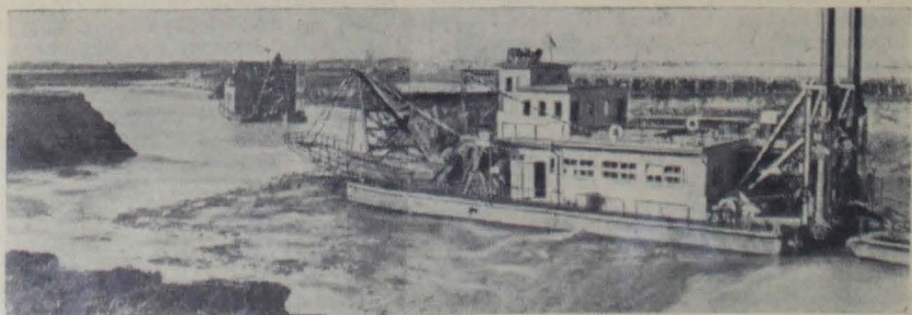
Сталинградгидрострой. Строители Сталинградской гидроэлектростанции закончили сооружение шестикилометрового Волго-Ахтубинского канала, продолженного через остров Зеленый. После разбора земснарядом последней перемычки шириной в 10 метров возлежние лоды пошли в Ахтубу по новому руслу.
