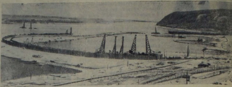
Куйбышевгидрострой. Строительство котлована под здание гидроэлектростанции. Фото Н. Фонинова. Прессклише ТАСС
