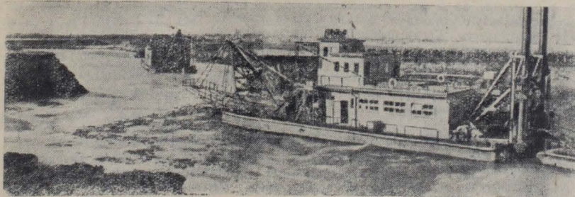
Сталинградгидрострой. Вид на Волго-Ахтубинский канал. Справа — земснаряд № 321.
