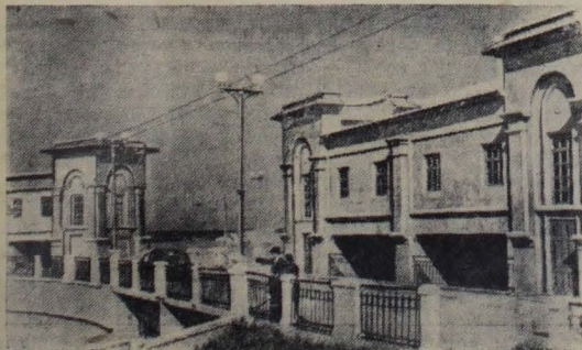
Ставропольский край. На строительстве Кубань-Егорлыкской оросительной системы. На снимке: головной шлюз Право-Егорлыкского канала. Фото Г. Аракеляна. Пресскляше ТАСС
