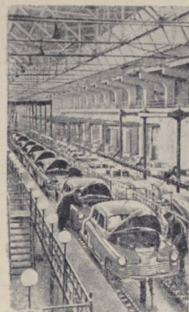
Горький. Эстакадный конвейер сборки автомобилей «Победа» на автозаводе имени В. М. Молотова. Фото П. Вознесенского.
