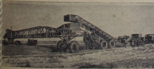
Парк машин и механизмов, действующих на строительных площадках гигантских гидроузлов и каналов, непрерывно пополняется новой техникой. На снимке: новая мощная машина — землеройный струг «Д-264», предназначенный для работы на строительстве судоходных и крупных магистральных оросительных каналов. Выпущенный стругом грунт разсыпается в сторону более чем на 45 метров. Машина движется с помощью трех тракторов «С-80». Опытный землеройный струг протестирован на строительстве канала Волга-Урал. Прессклиппе ТАСС
