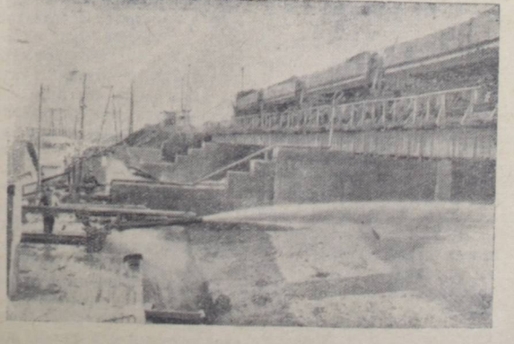
Азербайджанская ССР. В том месте, где многоводная Кура вливается в ущелье, образуемое утесами горного хребта Воя-Даг, сооружается Мингечаурская гидроэлектростанция. На снимке: размытый грунт гидромонитором в бундере-смесителе. Фото Ф. Шевцова.
