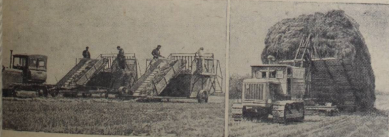
Ростовская область. Коллектив Всесоюзного научно-исследовательского института мелиорации и электрификации совхозов разработал высокопроизводительный комплекс сено- кожных машин. Эти машины за 8—10 часов обеспечивают комплексно-поточную уборку с 40—50 гектаров и повышают производительность труда, по сравнению со всеми дру- гим механизированными способами уборки сена, в 8—10 раз. В этом году новые машины применяются на уборке сена в колхозах и совхозах области.
