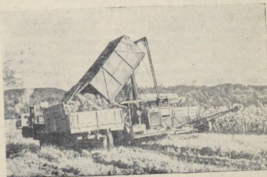
Хабаровский край. Для уборки силосных культур механизаторы Красноярского совхоза под руководством старшего агронома А. В. Михайленко переоборудовали выработанный зерновой комбайн «Коммунар» в силосный комбайн. Производительность его — до 15 тонн измельченной силосной массы в час.
