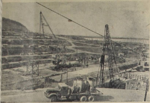
Куйбышевгидрострой. Общий вид работ в районе строительства лавана под здание ГЭС по Н. Финикова. Пресканише ТАСС
