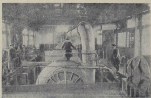
Куйбышевгидрострой. На великой стройке работает сверхмощный земснаряд «Сталинградский-1» — самый крупный в мире. Он может переместить за час тысячу кубометров грунта на расстояние до 4 километров.
