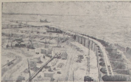
Каховский гидроузел. На участке сооружения продольной перемычки строители закончили забивку шпунта в ячейки. Замыть их ведется способом гидромеханизации. Земснаряд № 23 уже замыл пульпомассой более 15 ячеек. Одновременно идет укрепление берегового участка.
