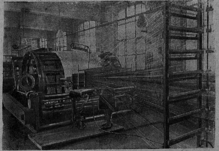
Шуйский машиностроительный завод имени Фрунзе выпускает для шелкоткацкой промышленности сновальную ленточную машину «СЛ-140 пл». Машина может вырабатывать от 40 до 300 метров основы в минуту. Ее производительность вдвое выше производительности машин прежних конструкций.
