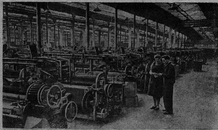
Московская область. На Егорьевском меланжевом комбинате за последние два года установлено более 500 высокопроизводительных автоматических станков отечественного производства. Это позволило значительно повысить выпуск продукции. В первом квартале коллектив комбината изготовил сверх плана 250 тысяч метров ткани. Во всех цехах развернулась борьба за дальнейшее повышение производительности труда, за досрочное выполнение годового плана. На снимке: ткацкий цех комбината. Фото И. Егорова. Прессклише ТАСС
