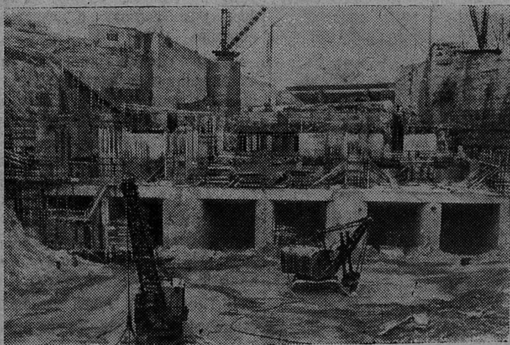
Эстонская ССР. Строительство здания Нарвской гидроэлектростанции. Фото В. Самусенко.
