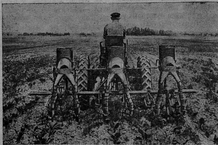
Культиватор-растениепитатель овощей „КРН-2,8“ к трактору „ХТЗ-7“.
