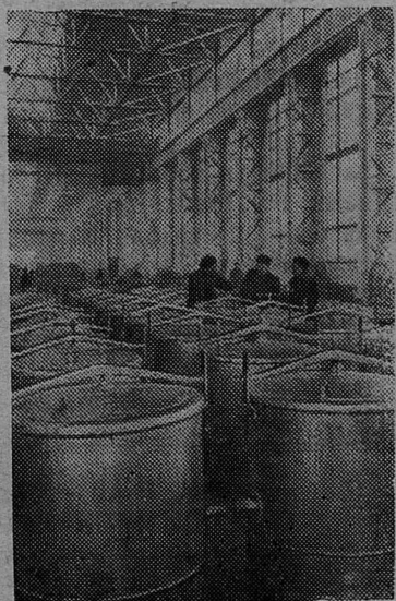
Алтайский край. Выполняя заказ сельского хозяйства, Барнаульский котельный завод освоил выпуск чанов для кормозапарников.
