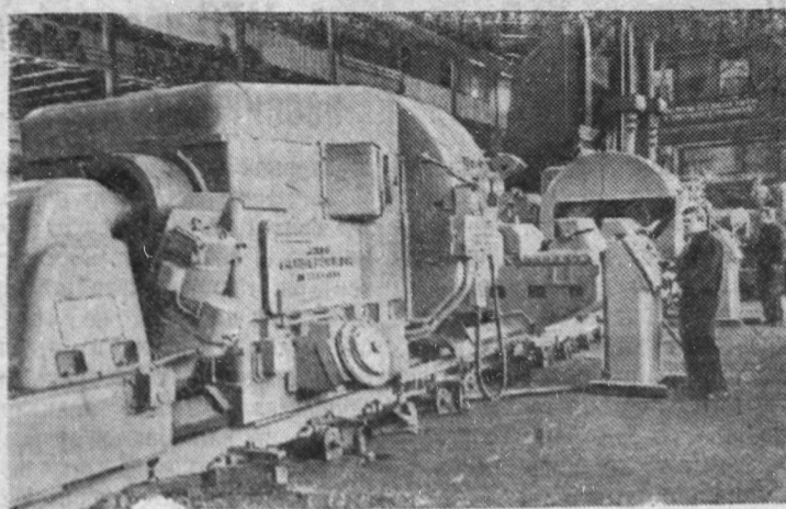
Ленинград. Завод имени Свердлова производит различные точные станки высокого класса точности. Недавно в сборочном цехе закончены испытания мощного расточного станка «ЛР-61», предназначенного для обработки турбинных доплаток. Станок оснащен 26 электромоторами, имеет два пульта управления и обслуживается одним человеком.
