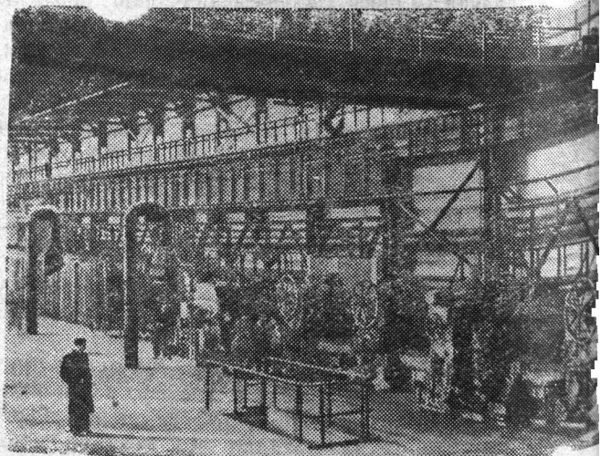
На Челябинском металлургическом заводе закончилось строительство нового прокатного стана „300“. Он будет выпускать новое прокат мелкого профиля и арматурное железо. Стан построен по последнему слову техники. Управление его узлами полностью механизировано и автоматизировано. В отличие от других в этом стане имеется одна большая нагревательная печь, вместо двух. На снимке: общий вид стана „300“. Фото В. Георгиева.
