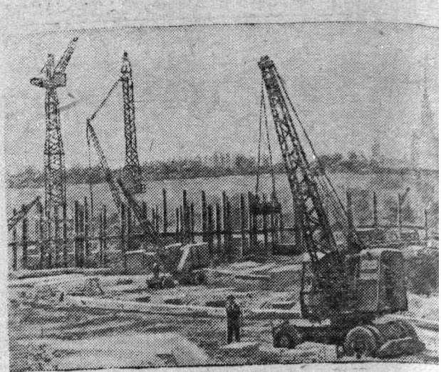
Москва. В Лужниках, на месте бывших пустырей развернулось строительство нового столичного стадиона. Объем работ предстоит выполнить строителям спортивно-технической тресту «Ленспецстрой». Только на трибуны главной арены пойдет свыше сорока тысяч стальных конструкций. Здесь будет уложено сорок миллионов штук кирпича и более 20 тысяч кубометров бетона. На снимке: на строительстве стадиона в Лужниках. Фото В. Кошерева.
