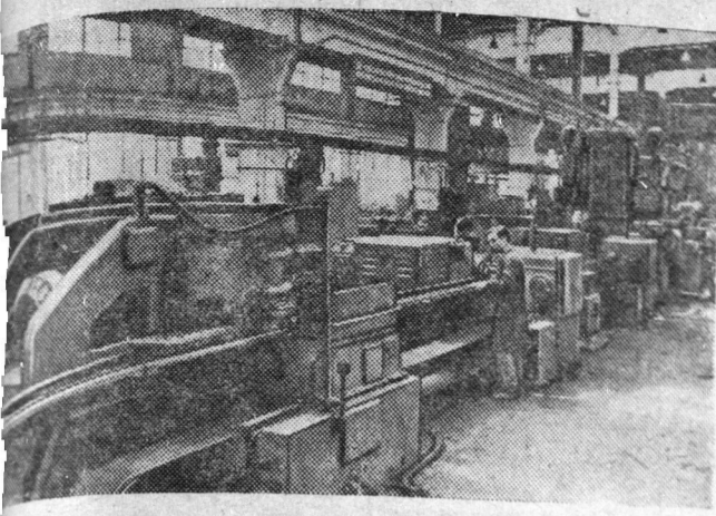
Московский станкостроительный завод имени Серго Орджоникидзе начал выпускать более ста агрегатных станков новой конструкции. Коллектив сборщиков раньше срока закончил сборку станка новой автоматической линии, предназначенной для обработки головок блока цилиндров трактора «ДТ-54». На снимке: новая автоматическая линия, изготовленная заво-
