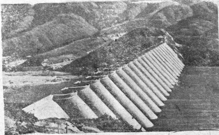
Фоззалинское водохранилище на реке Бихэ (провинция Аньхуэй). Его емкость — 470 миллионов кубических метров воды.
