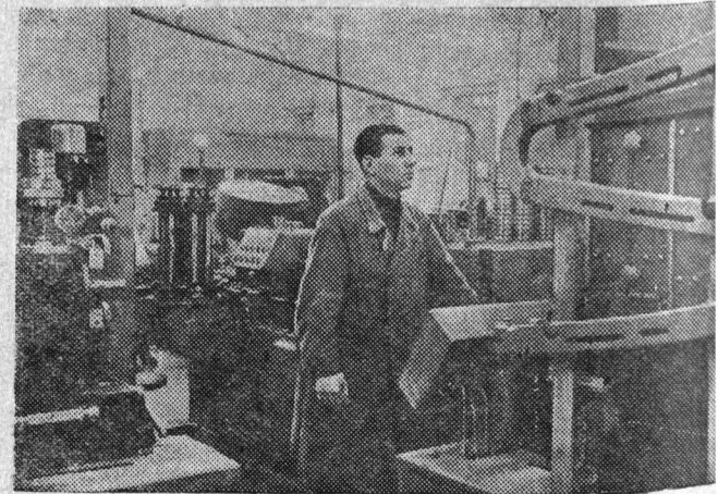
Москва. На Первом подшипниковом заводе имени Л. М. Вича технические комиссии принимают в эксплуатацию автоматическую линию цеха массовых подшипников.
