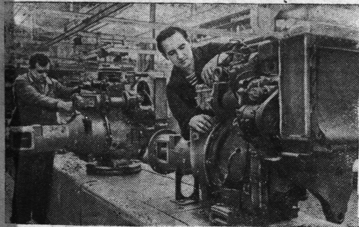
Харьковский тракторный завод освоил выпуск пропашных тракторов «ДТ-14» с дизельным двигателем. На снимке: конвейер сборки дизельных моторов к трактору «ДТ-14». Справа — слесарь Александр Ерохин, выполняющий норму на 150 и более процентов.
