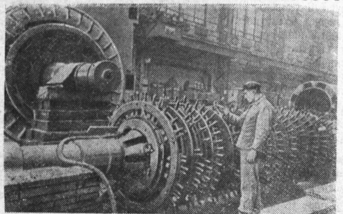
Соревнуясь за достойную встречу XX съезда КПСС, коллективы заводов и фабрик Ленинграда стремятся ознаменовать 1956 год новыми трудовыми успехами. Коллектив турбокорпуса завода «Электросила» имени С. М. Кирова в начале года выпустил несколько мощных генераторов. На снимке: обмотчик коммунист А. И. Тепляков проверяет температуру при запечке ротора турбогенератора мощностью в 50 тысяч киловатт. Фото А. Михайлова.
