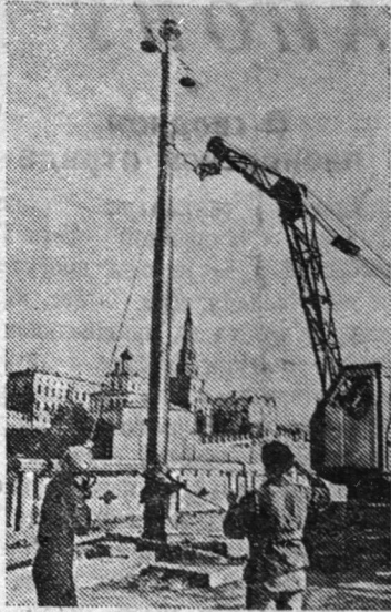
Казань. В связи с созданием Куйбышевского водохранилища уровень Волги у Казани поднимется. Сейчас в городе ведутся работы, связанные с его защитой от опасности наводнения. Уже готов железнодорожный мост. Закачивается строительство транспортного моста. На снимке: установка металлических столбов освещения на новом транспортном мосту у Казанского кремля.
