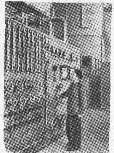
На Макеевском металлургическом заводе имени Кирова построена новая кислородная станция. Станция будет давать кислород сталеплавильщикам первого мартеновского цеха. Применение кислорода на всех печах цеха даст возможность увеличить выплавку стали больше чем на двадцать процентов. НА СНИМКЕ: сменный инженер В. В. Денисов у пульта управления.
