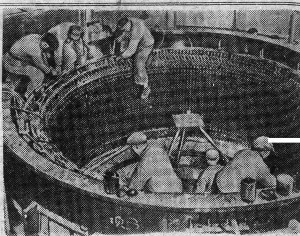
Китайская Народная Республика. На реке Юнди ружается первая в Северном Китае Гуаньтинская гидроэлектростанция. Сейчас ведется монтаж оборудования. Станция электростанции будет завершена в 1956 году. Гидроэлектростанция даст дополнительную энергию вольтовой линии, связывающей города Пекин, Тяньцзинь и Калган.
