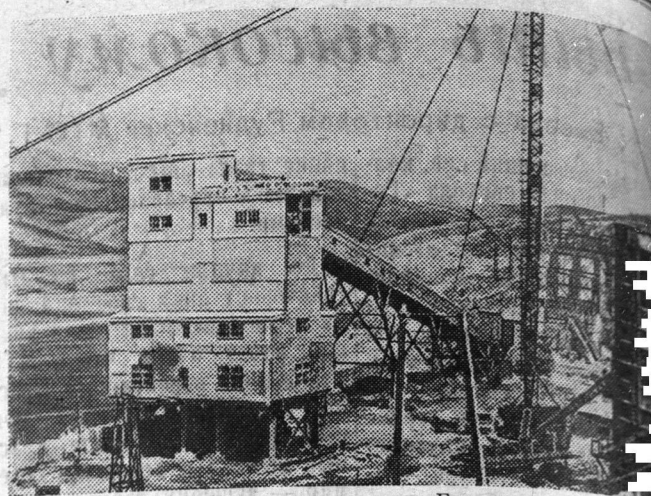
Казахская ССР. На строительстве Бухтарминской ГЭС. На снимке: бетонный завод. Фото А. Бахвалова.
