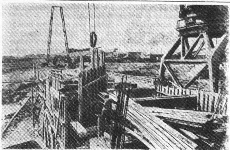
Новосибирская область. В будущем году должна дать промышленный ток первая очередь Новосибирской ГЭС. Зимой будет перекрыто русло Оби. Чтобы обеспечить своевременный пуск основных сооружений гидроузла, строители должны проделать огромную работу по укладке бетона, намыву грунта, монтажу металлоконструкций. Развернулось соревнование с коллективом строителей Иркутской ГЭС за досрочное выполнение плана первого года шестой пятилетки.
