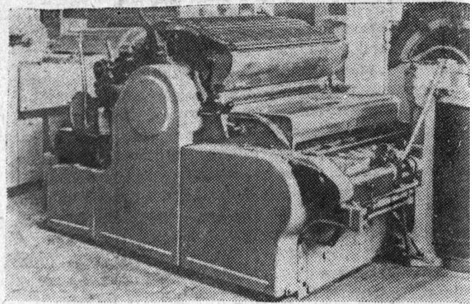
На снимке: чесальная малогабаритная машина ЧММ-450, голенная ленинградским заводом «Вулкан».
