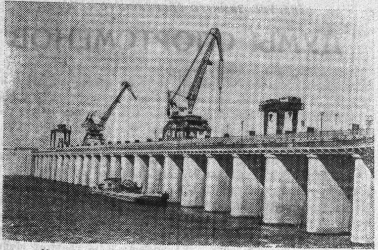
Новая Наховка. Плотина Каховского гидроузла.
