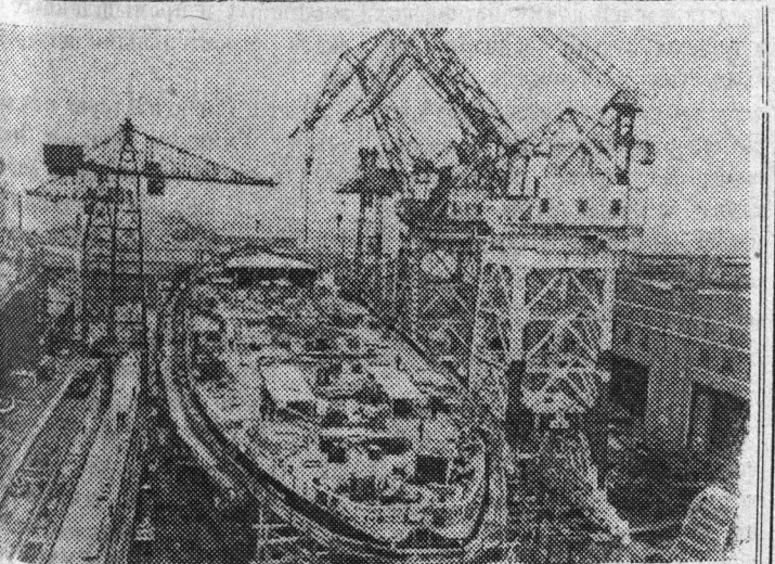
Ленинград. На строительстве атомного ледокола «Ленин». На снимке: общий вид строительства ледокола. Фотохроника ТАСС
