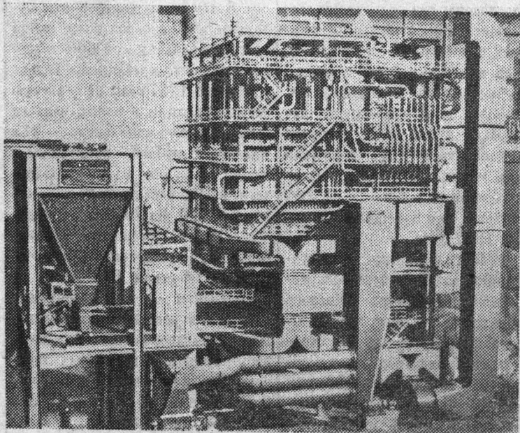
На снимке: макет прямого котла-гиганта.
