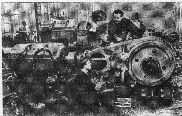
Коллектив Металлического завода получил заказ изготовить две напольно-завалочные машины для строящегося металлургического комбината в Китае. Сборка машин идет успешно.
