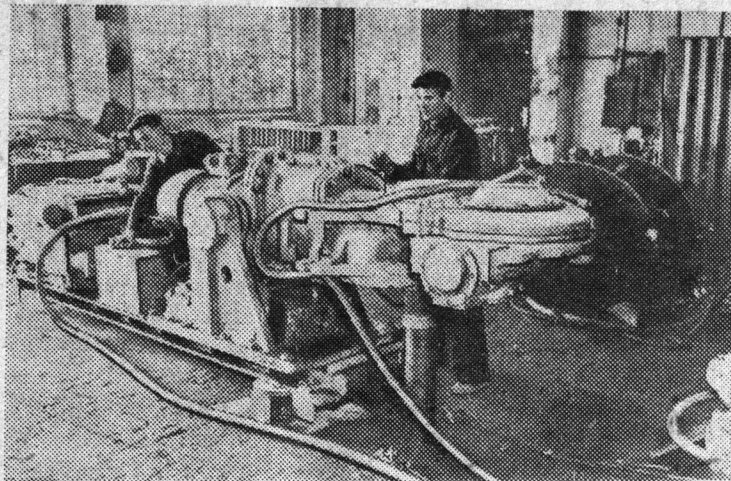
Челябинская область. На Копейском заводе горного машиностроения имени Кирова изготовлен опытный экземпляр нового угледобывающего комбайна «Урал-2». При его конструировании учтены условия добычи топлива на шахтах области.
