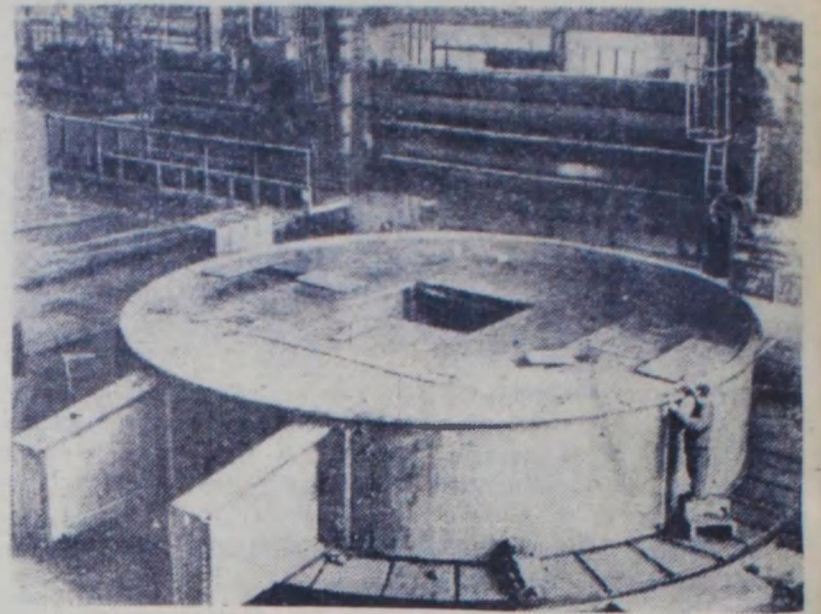
Чехословацкая Республика. На заводе имени Клемента Готвальда в Витковичах создается мощный отвалообразователь. Эта машина предназначена для размещения горных пород на отвалах в открытых угольных разработках имени Яна Швермы. Машина сможет отваливать за час до 1.800 кубометров породы и транспортировать ее на расстояние до 70 метров. Отвалообразователь обслуживается пятью рабочими.
