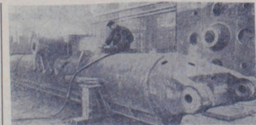
Коллективу Ижорского завода поручено в этом году осво-ить производство 19 новых типов машин и механизмов. Неко-торые из них уже созданы. Сейчас в сборочном цехе идет об-работка деталей модели «ЭК 8».
