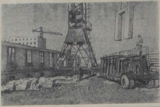
Ленинград. УНР 63 треста № 102 Главленинградстрой на сооружении корпуса № 12 в 67-м квартале Московского района применил, по примеру московских строителей, монтаж крупных блоков прямо с блоквоза. Это значительно ускоряет процесс монтажных работ. На снимке: монтаж новым методом. Слева корпус через 12 часов после начала монтажа 1-го этажа. ЛенТАСС
