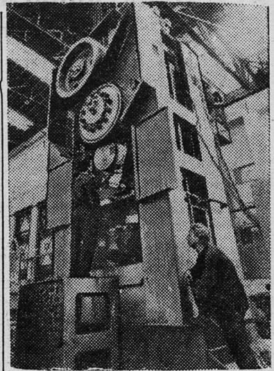
Чехословацкая Республика. На машиностроительном заводе имени Б. Шмерала в Брно сооружается вертикальный кузнечный пресс ЛКМ-1600, который будет выставлен на Первой международной ярмарке в сентябре 1959 года в Брно. На снимке: вертикальный кузнечный пресс. Фото Э. Бицана. Чехословацкое телеграфное агентство
