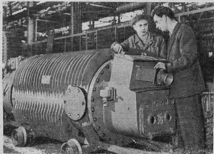
Украинская ССР. Запорожский трансформаторный завод изготовил для угольных шахт взрывобезопасную трансформаторную подстанцию мощностью 180 киловольт-ампер на напряжение 6 киловольт.
