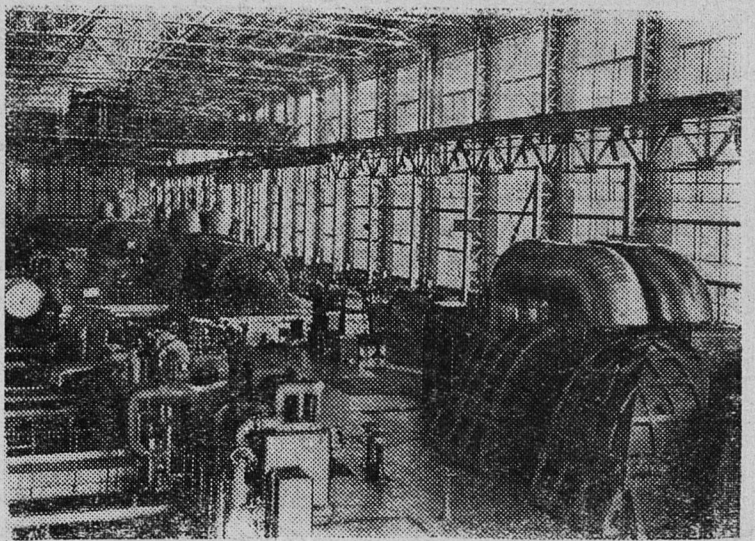
СТАЛИНСКАЯ ОБЛАСТЬ. Закончен монтаж и начато опробование еще одного турбогенератора на строящейся Старобшевской ГРЭС. Тем самым завершено сооружение первой очереди этой крупной тепловой электростанции. Ее первые агре-
