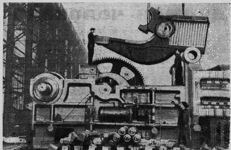
Сталинская область. На стенде механического цеха № 7 Ново-Краматорского завода идет сборка новой горизонтально-ковочной машины давлением 3.150 тонн. Этот мощный агрегат будет производить штамповку колец для подшипников качения.
