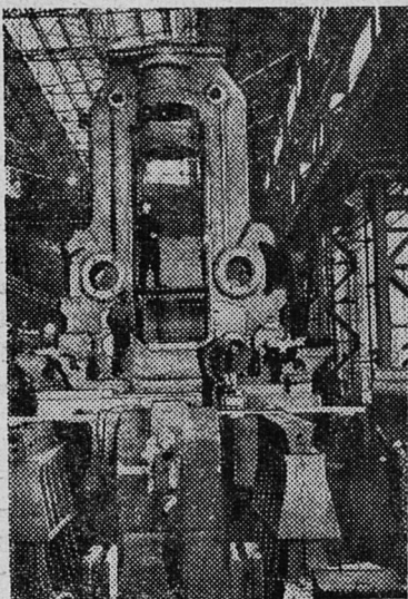
Свердловск. В цехах Уральского завода тяжелого машиностроения изготавливается гигантский рельсобалочный стан. На снимке: обжимная рабочая клеть. Фотохроника ТАСС
